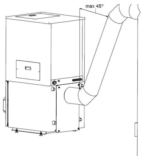
Rysunek 15 - Podłączenie do instalacji kominowej – pochylone 1 – Przewód kominowy; 2 – Wyczystka kominą; 3 – Zaizolowane podłączenie do kominą
