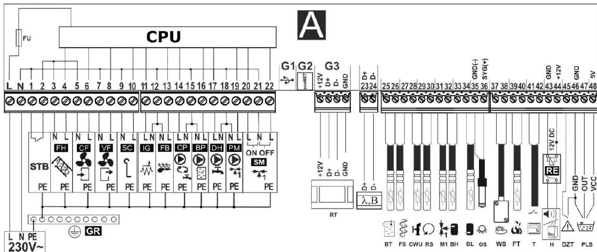
Rysunek 22 - Schemat połączeń elektrycznych regulatora
