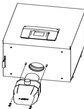
Rysunek 12 - Montaż palnika
