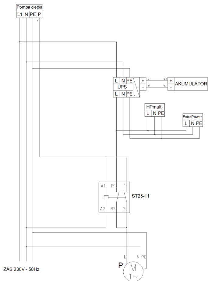
b) schemat elektryczny dla układu 1 - fazowego
