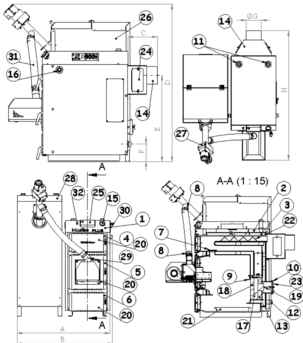
Rys. 2B Wymiary i opis kotła MASTER PLUS opcja zbiornik z boku.
