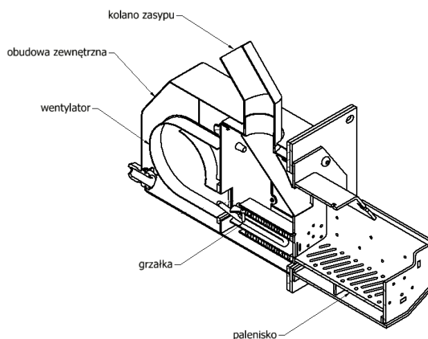
Rys. 5 Budowa palnika
