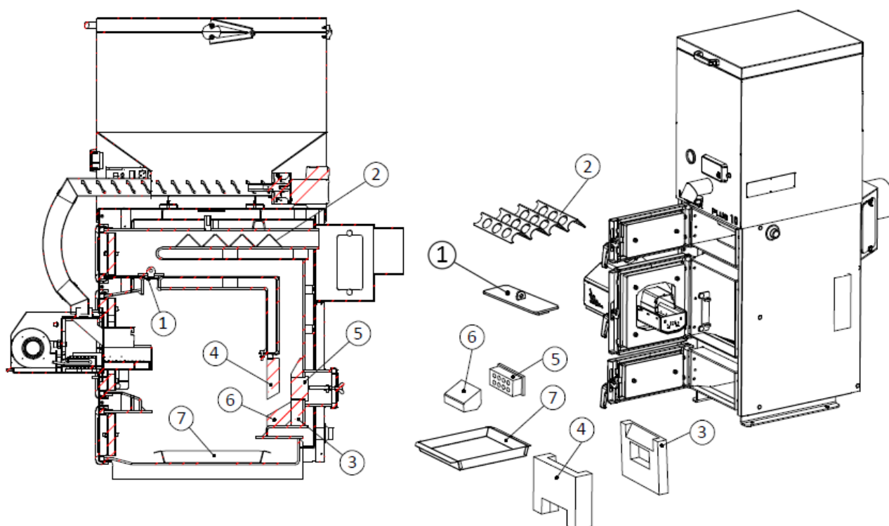
Rys. 18 Lokalizacja płyt szamotowych w kotle Master, Master Plus
