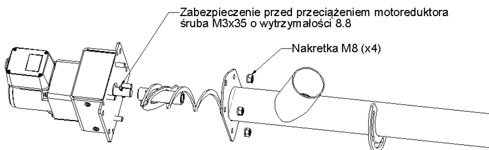
Rys. 7 Montaż podajnika śrubowego (opcja z zbiornikiem u boku)
