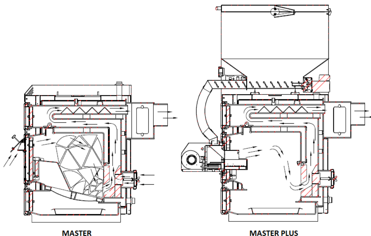
Rys. 16 Schemat obiegu spalin dla kotła Master i Master Plus - efektywna praca
