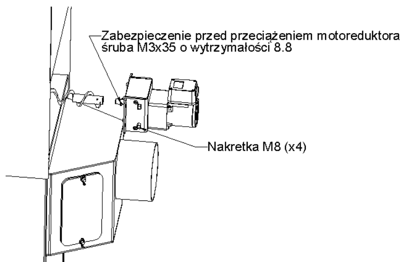
Rys. 6 Montaż podajnika śrubowego (opcja z zbiornikiem u góry)
