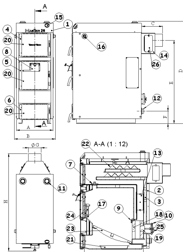
Rys. 1B Wymiary i opis kotła MASTER o mocy 22, 26 kW z zasypem ręcznym
