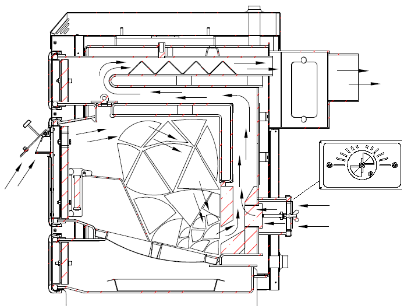
Rys.13 Długi obieg spalin - praca efektywna kotła Master
