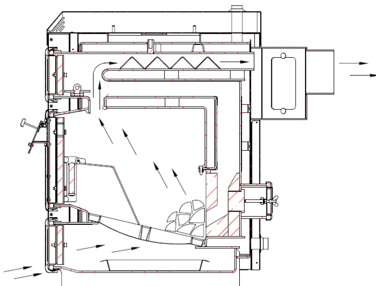
Rys. 12 Krótki obieg spalin – rozpalanie i napełnianie komory paliwem kotła Master.
