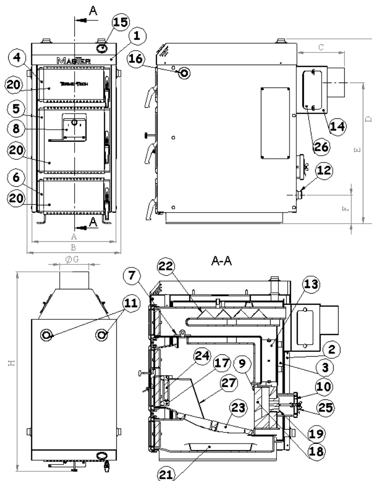
Rys. 1A Wymiary i opis kotła MASTER o mocy 10, 15 kW z zasypem ręcznym
