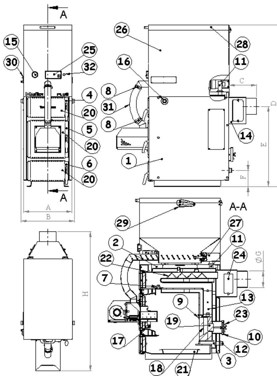
Rys. 2A Wymiary i opis kotła MASTER PLUS opcja zbiornik u góry
