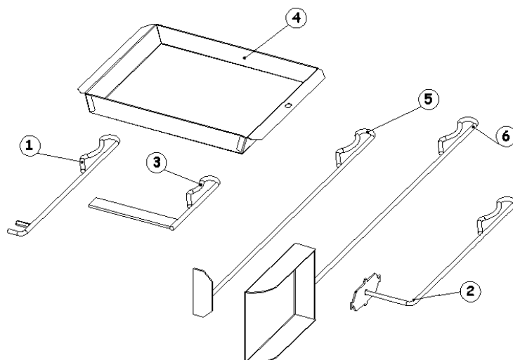
Rys.14 Uchwyty do obsługi i czyszczenia kotła.
